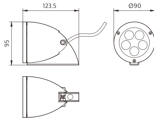
BGP312 LED5
